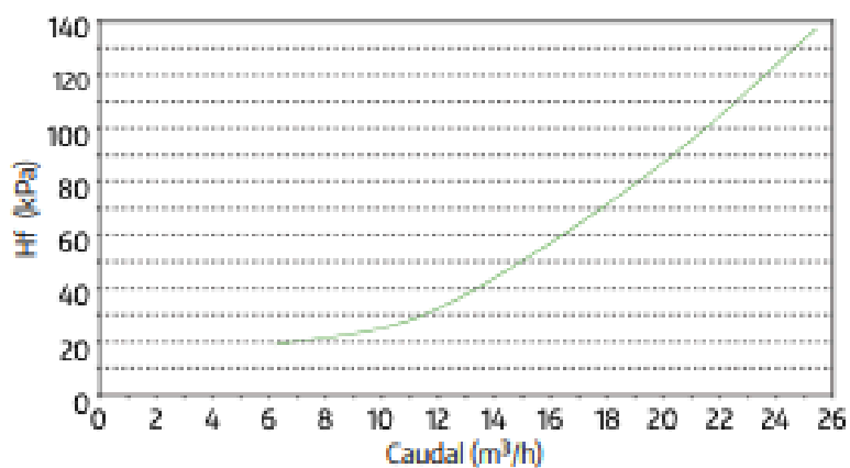
Perda de Carga - Válvula 1 1/2"
