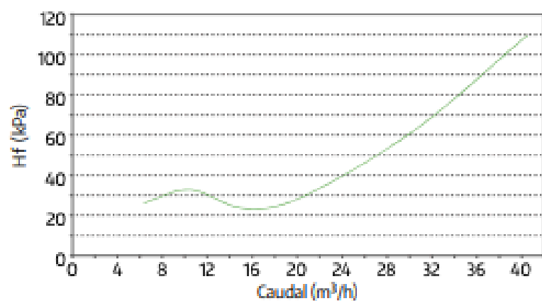
Perda de Carga - Válvula 2"
