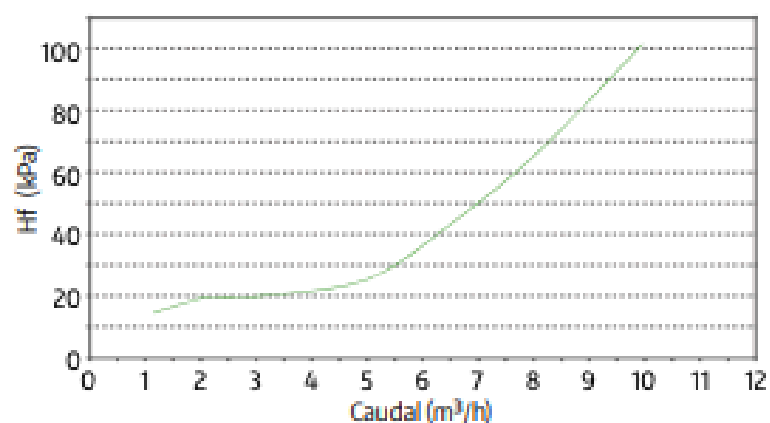
Perda de Carga - Válvula 1"
